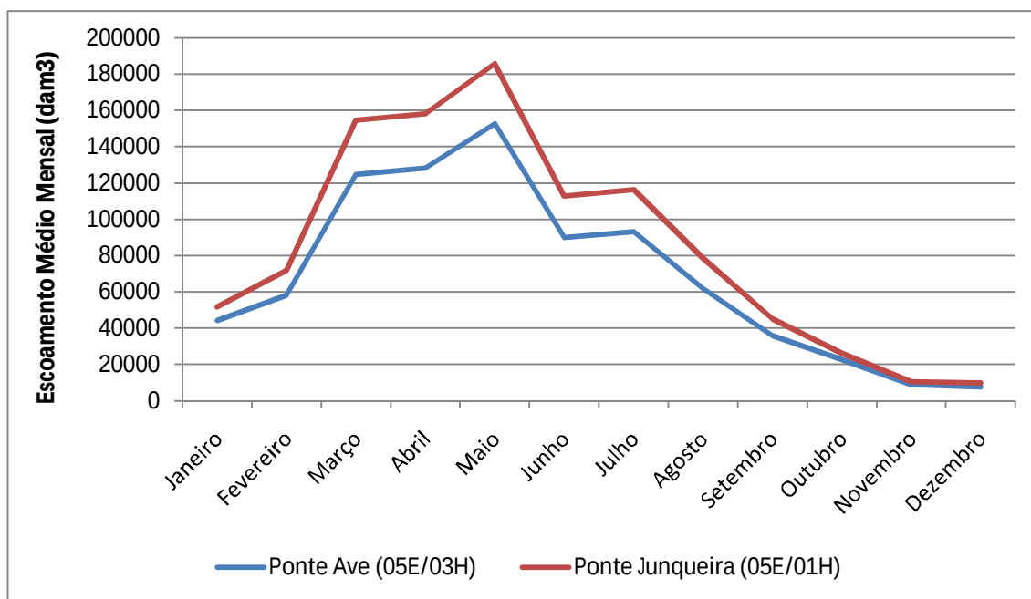
Figura 4.28 – Variação do escoamento médio mensal nas estações consideradas
