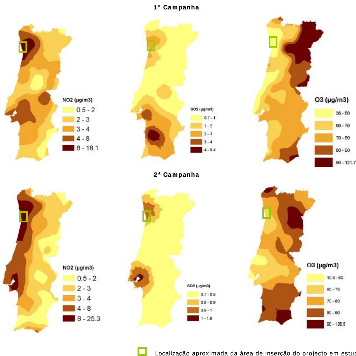
Figura 4.44 - Curvas de isoconcentrações de dióxido de azoto, dióxido de enxofre e ozono no ar ambiente em Portugal Continental
