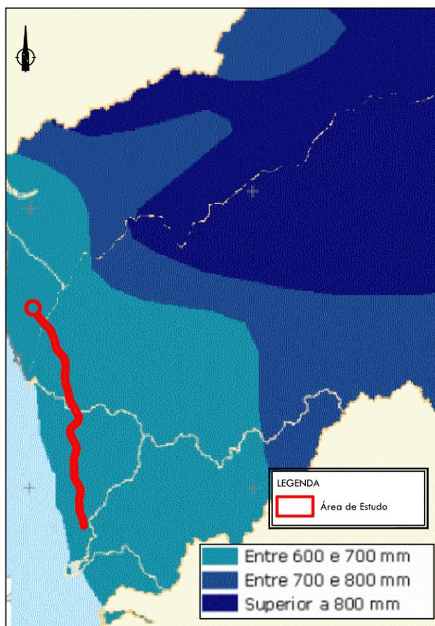
Figura 4.26 – Escoamento – Valores Médios Anuais (mm)
