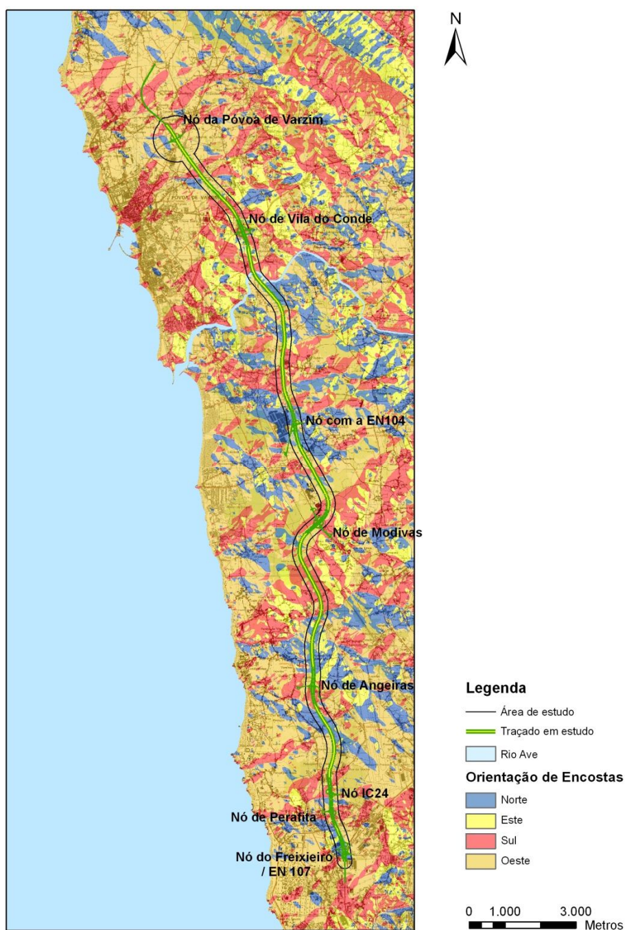
Figura 4.77 – Carta de Orientações das encostas
