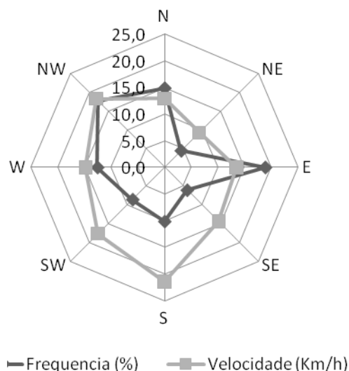
Figura 4.42 – Frequência e Velocidade média anual do vento registadas na Estação Climatológica de Porto/Pedras Rubras
